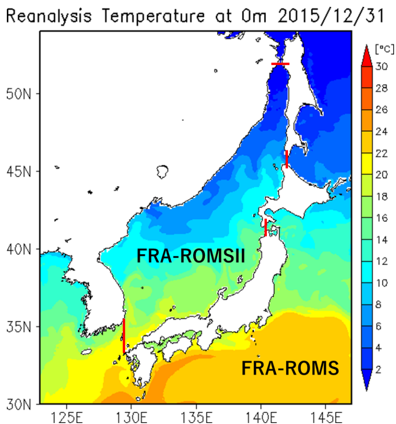
図 1 : 2015 年 12 月 31 日の再解析値水温. FRA-ROMS と FRA-ROMSII のデータの境界を赤線で示す。
